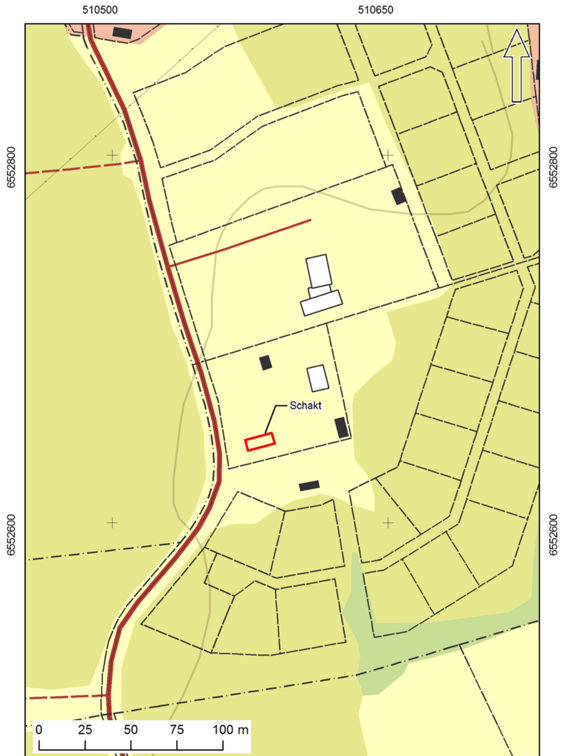
Figur 5. Schaktplan. Skala 1:2 000.
