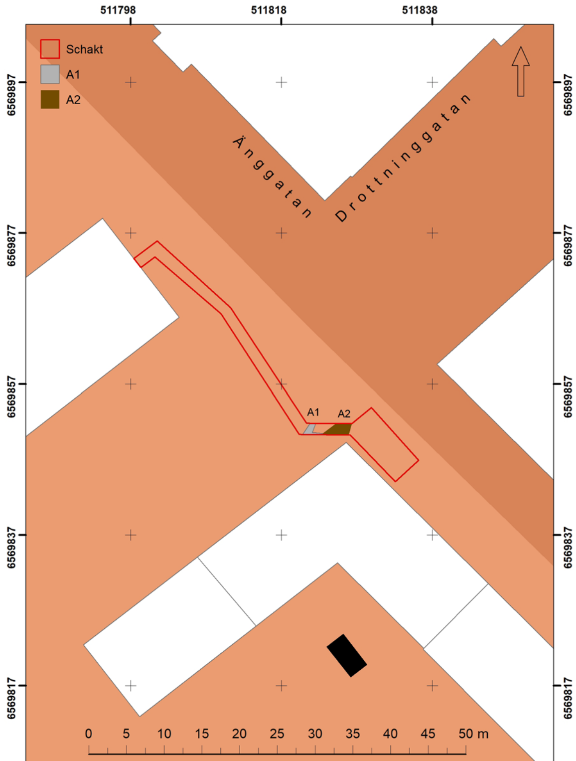
Figur 3. Schakt- och anläggningsplan. Skala 1:500.
