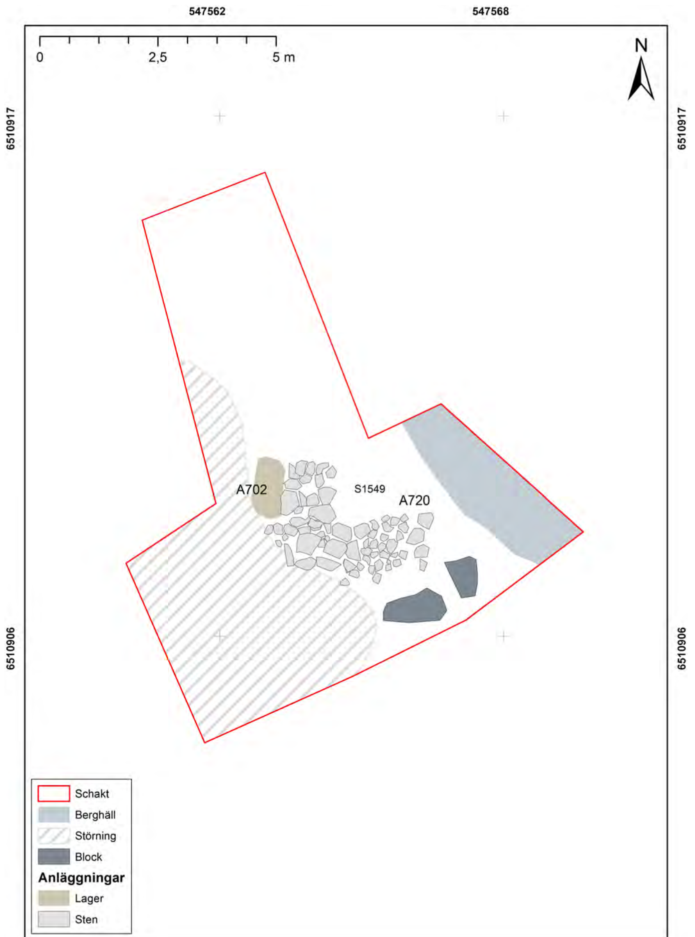
Figur 22. Plan över konstruktionen A720. Skala 1:80.
