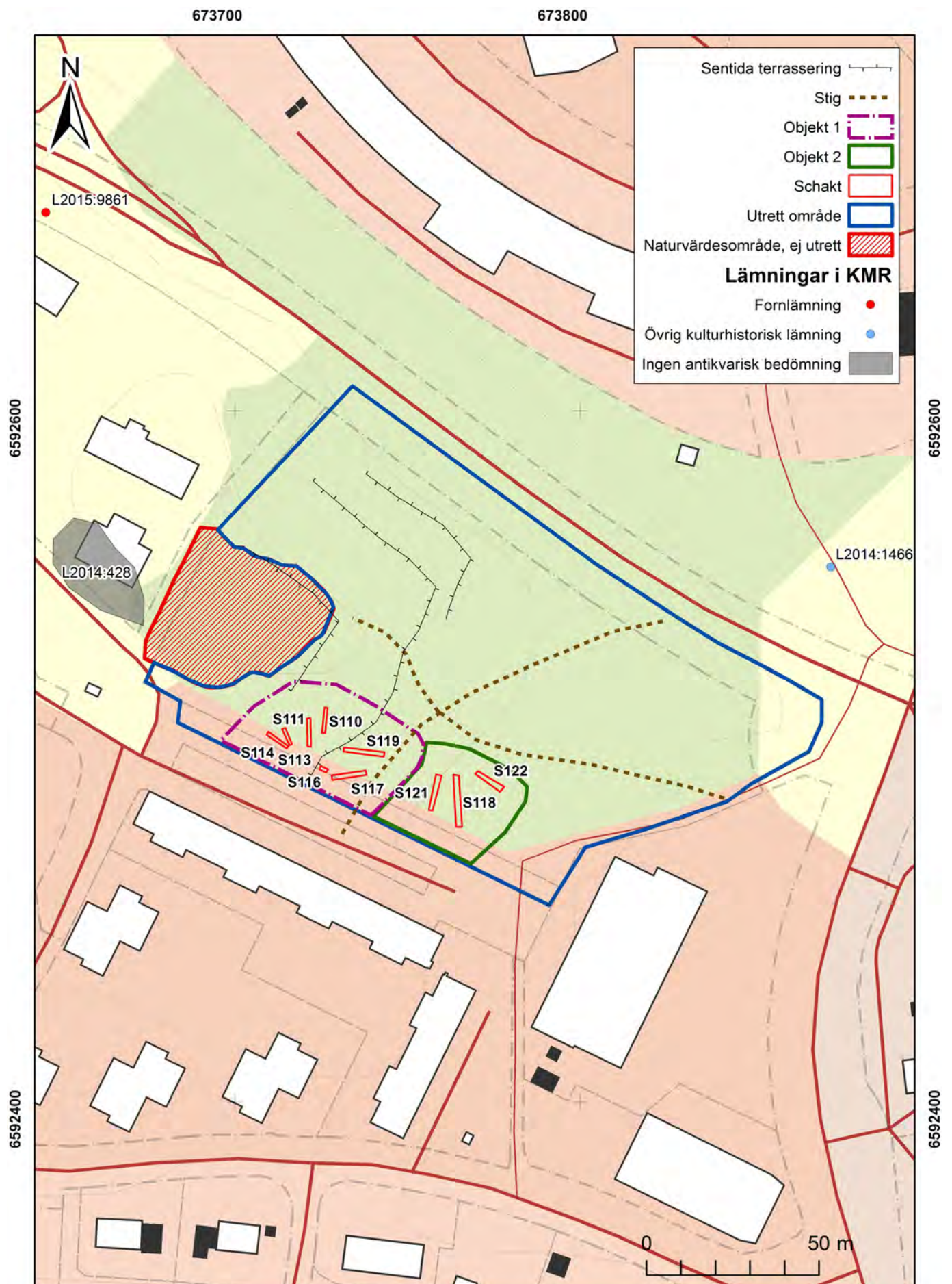
Figur 10. Schaktplan. Skala 1:1 500.
